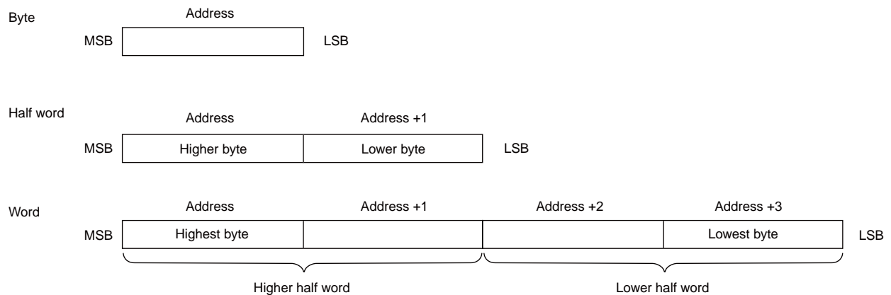
Figure 2.2-4 Big Endian Byte Orde
