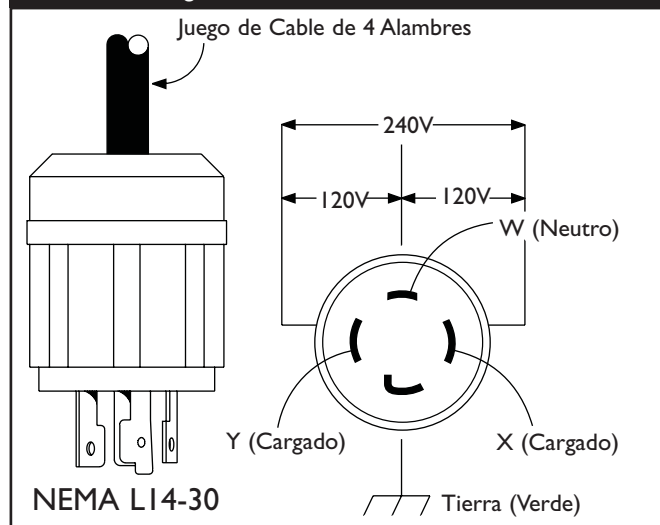
Figura 12 — 120/240 Volt AC, 30 Amp, Receptáculo de Seguridad
