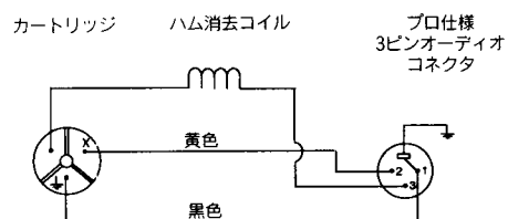
内部接続図
