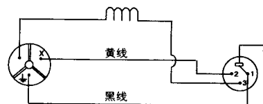
内部连接
