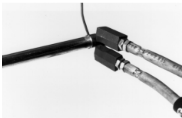
Figura 7 – Soldadura con las puntas de carbono sólo en contacto con el fitting
