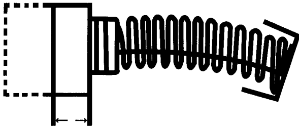
Figura 10 – Desgaste de una escobilla de carbono
