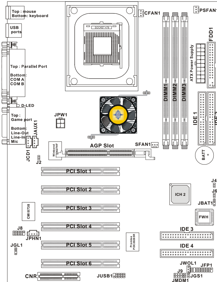
845 Pro2-R (MS-6528 v1.X) ATX Mainboard
