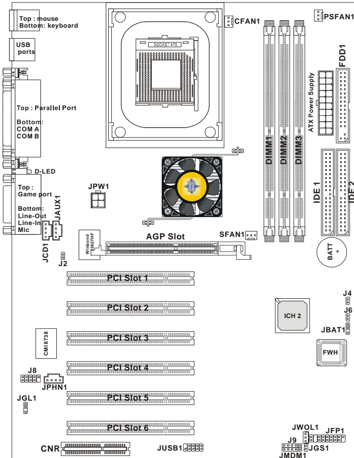
845 Pro2 (MS-6528 v1.X) ATX Mainboard
